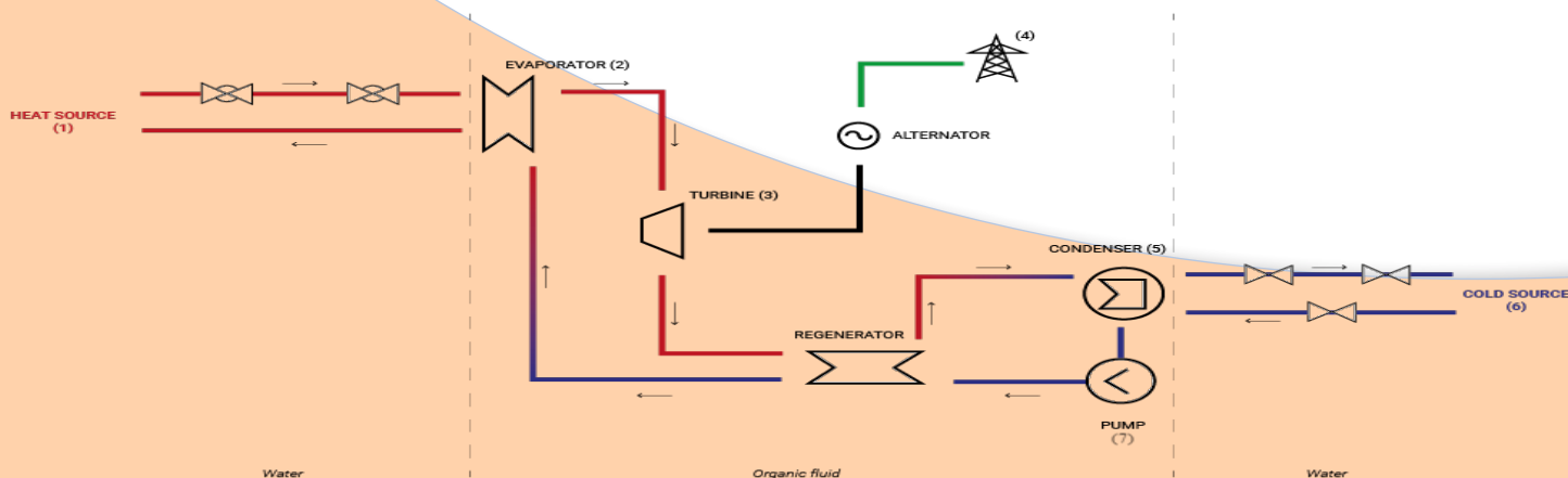
Figure 1 - Funzionamento ORC
